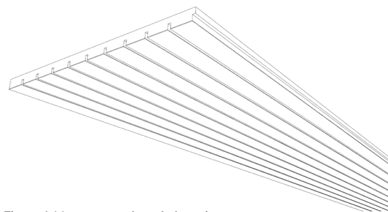
• Figure 1. Vue en coupe isométrique du panneau STRATA 1903.
