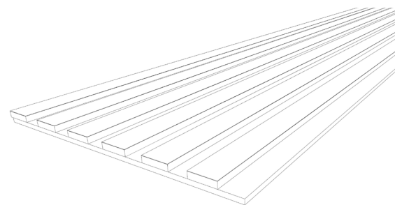
Figure 6. Vue en coupe isométrique du panneau acoustique HARMONY 5136.
