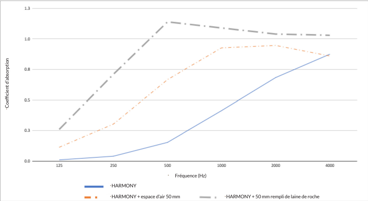
Figure 1. Performances acoustiques du panneau HARMONY 2713.
